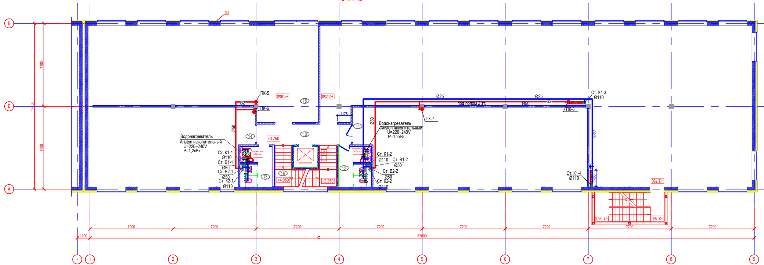
План 2-го этажа с системами В1; Т3; К1; К2
